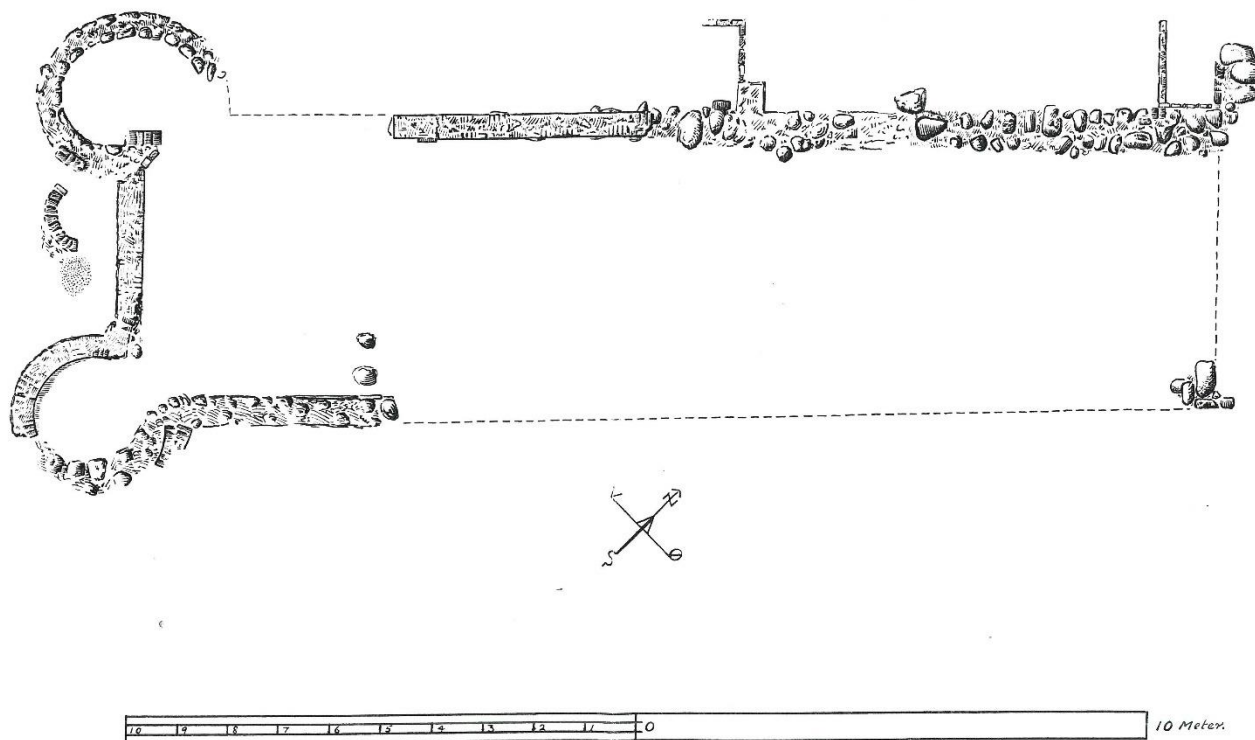
Fundamentsrester fra Frydenborg opmålt af S. A. Claudi-Hansen efter udgravningen 1911.
